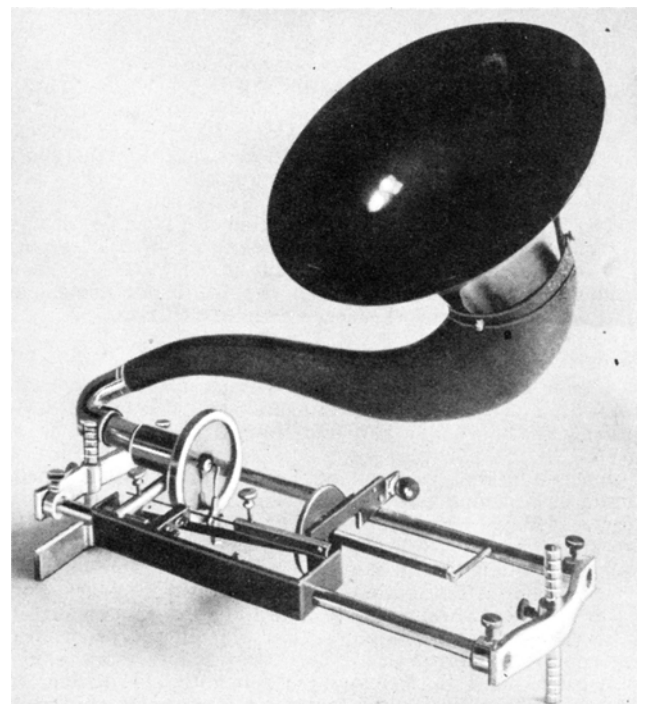
So fing die Schallplatten-Selbstaufnahme einmal an: Eines der ersten akustischen Selbstaufnahmegeräte mit Trichter und Aufnahmedose mit Glimmermembran. (Archivbild)
