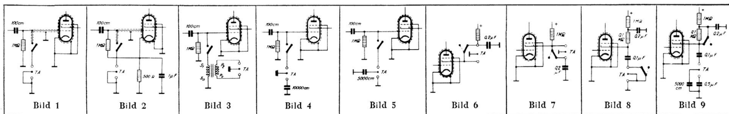
Bild 1: Gebräuchliche Anschaltung des Tonabnehmers TA an das Steuergitter eines Audions (für Wechselstrom und Batterie). Bild 2: Hier erhält das Fünfpolaudion bei Schallplattenwiedergabe eine kleine negative Vorspannung. Bild 3: Ein Niederfrequenztransformator ist bei schwachem Niederfrequenzteil vorteilhaft, er riegelt außerdem den Tonabnehmer völlig vom Netz ab (für Allstrom besonders geeignet). Die Abschirmung der Tonabnehmerschnur wird unmittelbar geerdet. Bild 4: Abriegelung des Tonabnehmers durch einen durchschlagsicheren Block von 10 000 pF (für Allstromgeräte). Abschirmung wird ebenfalls unmittelbar geerdet. Bild 5: Neue Schaltung für Allstromempfänger.. Der Tonabnehmer ist mit einem Netzpol unmittelbar verbunden. Beste Berührungssicherheit Vorbedingung! Bild 6: Anschaltung des Tonabnehmers ans Schirmgitter eines Fünfpolaudions (nur bei zeitgemäßer Endröhre möglich). Der Schalterkontakt schließt den
