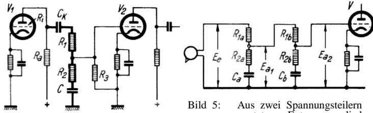
Bild 4: Einfügung der Baßanhebung zwischen Anoden- und Gitterkreis zweier Verstärkerstufen V_1 und V_2 . R_a = Anodenwiderstand, C_k = Kopplungskondensator = 20000-30000 pF, R_3 = Gitterableitwiderstand = 1 bis 2 M \Omega , R_1 = 0,3M \Omega , R_2 = 53k \Omega , C = 18000 \mu F, f_1 = 30, f_2 = 200.
